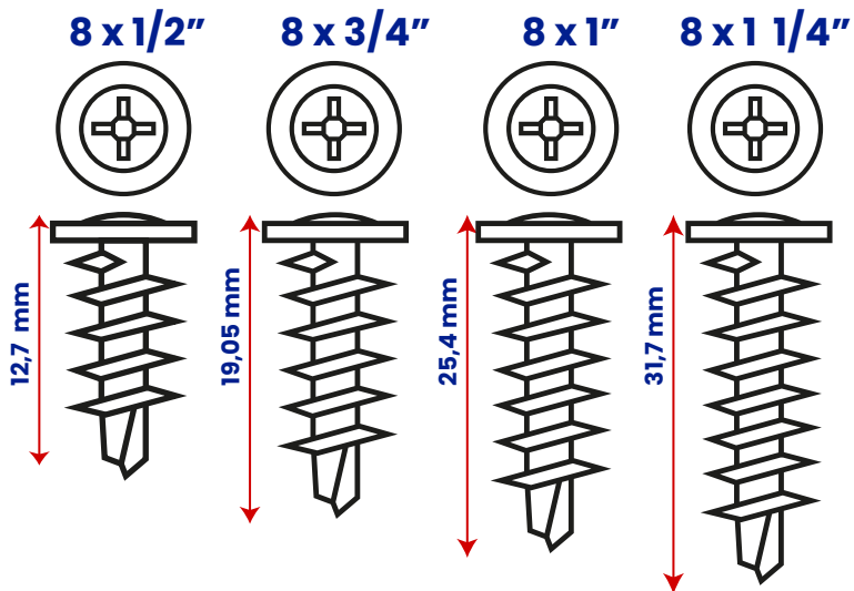
MATERIAL:ACERO ZINCADO
